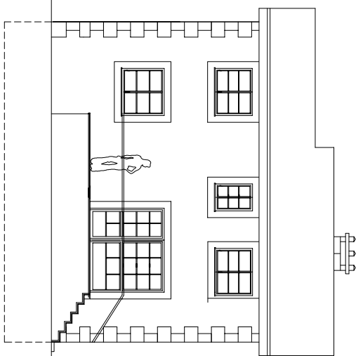
ALZADO NORTE
