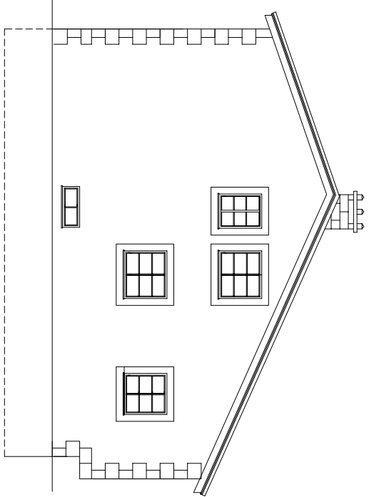
ALZADO OESTE
